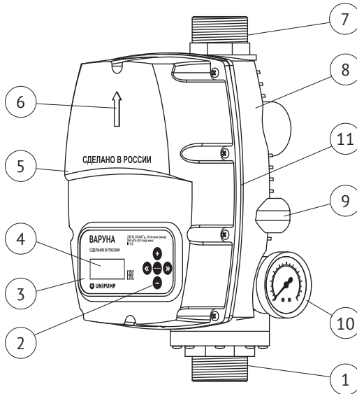
Рис. 1. Общее устройство
